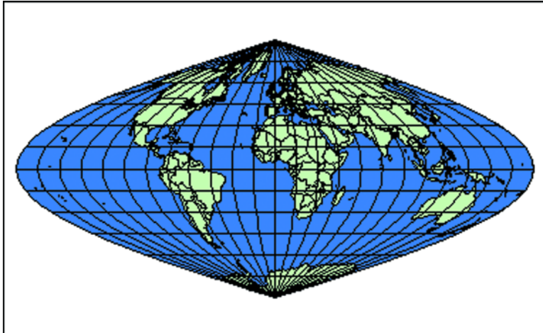
Sinusoidal (Equal-Area)
